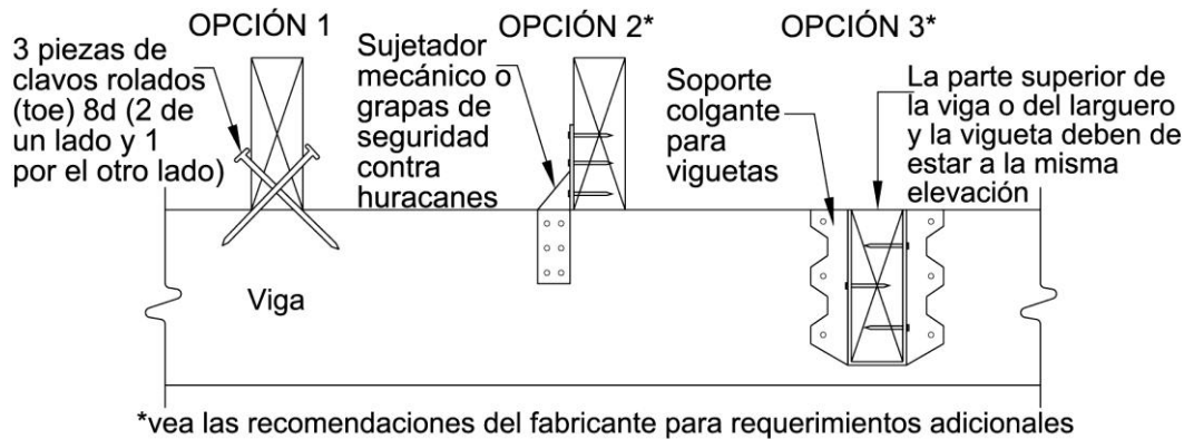
Figura 6. Detalle Vigueta-a-Viga.
