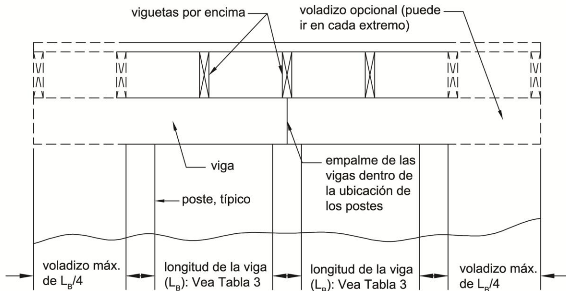
Figura 3. Longitudes de Vigas.
