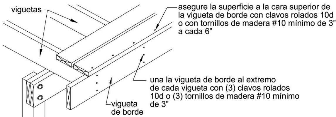
Figura 11. Detalles de Conexión de Vigueta de Borde.
