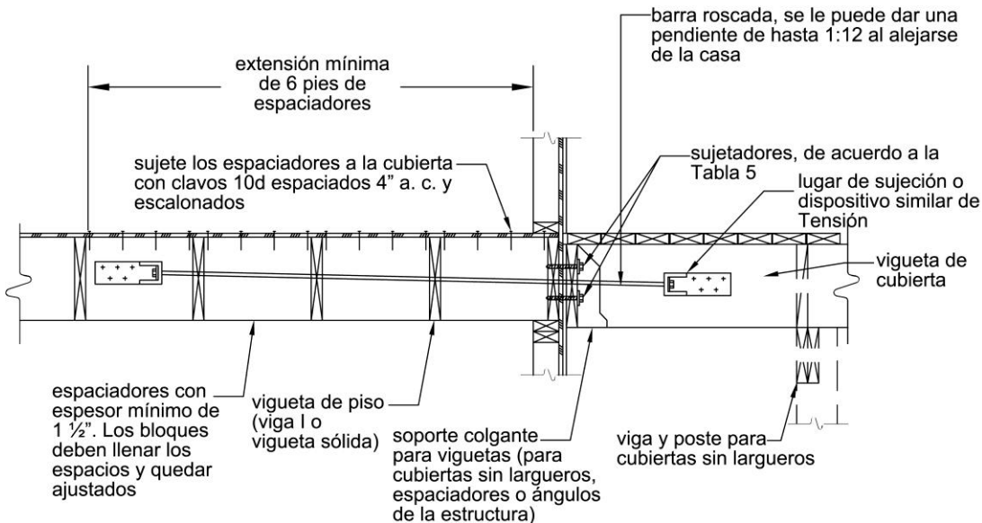
Figura 23. Dispositivo de Carga Lateral con Viguetas Perpendiculares a las Viguetas de la Cubierta.
