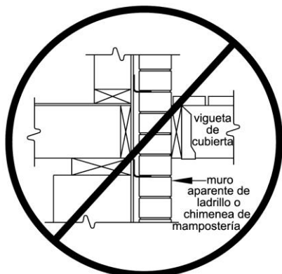
Figura 17. No unir a muros exteriores aparentes ni atravesarlos (ladrillo, mampostería o piedra).
