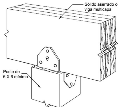
Figura 9. Condición de Unión Prohibida Poste-a-Viga.
