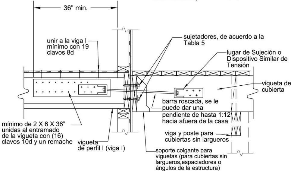
Figura 23. Dispositivo de Carga Lateral con Viguetas Perpendiculares a las Viguetas de la Cubierta.
