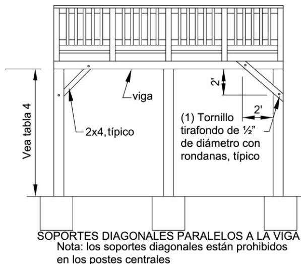
Figura 10. Soportes Diagonales.
