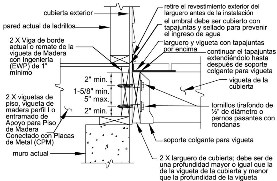
Figura 14. Unión General de la Tabla del Larguero a la Viga del Borde o Remate de la Vigueta.
